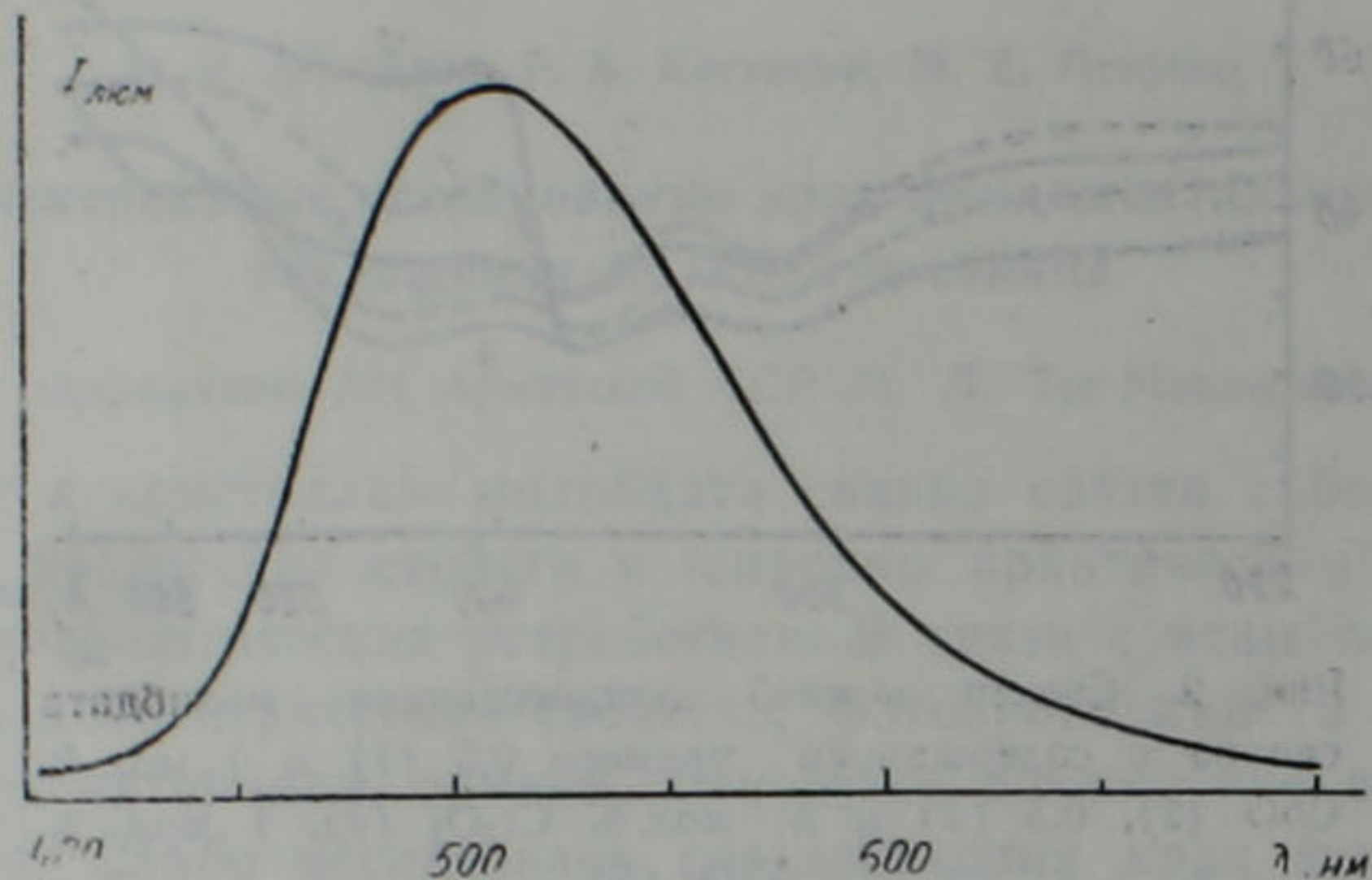
Рис. 2. Спектр зеленой люминесценции молибдата свинца с содержанием 1 мол. % \text{CoO}
