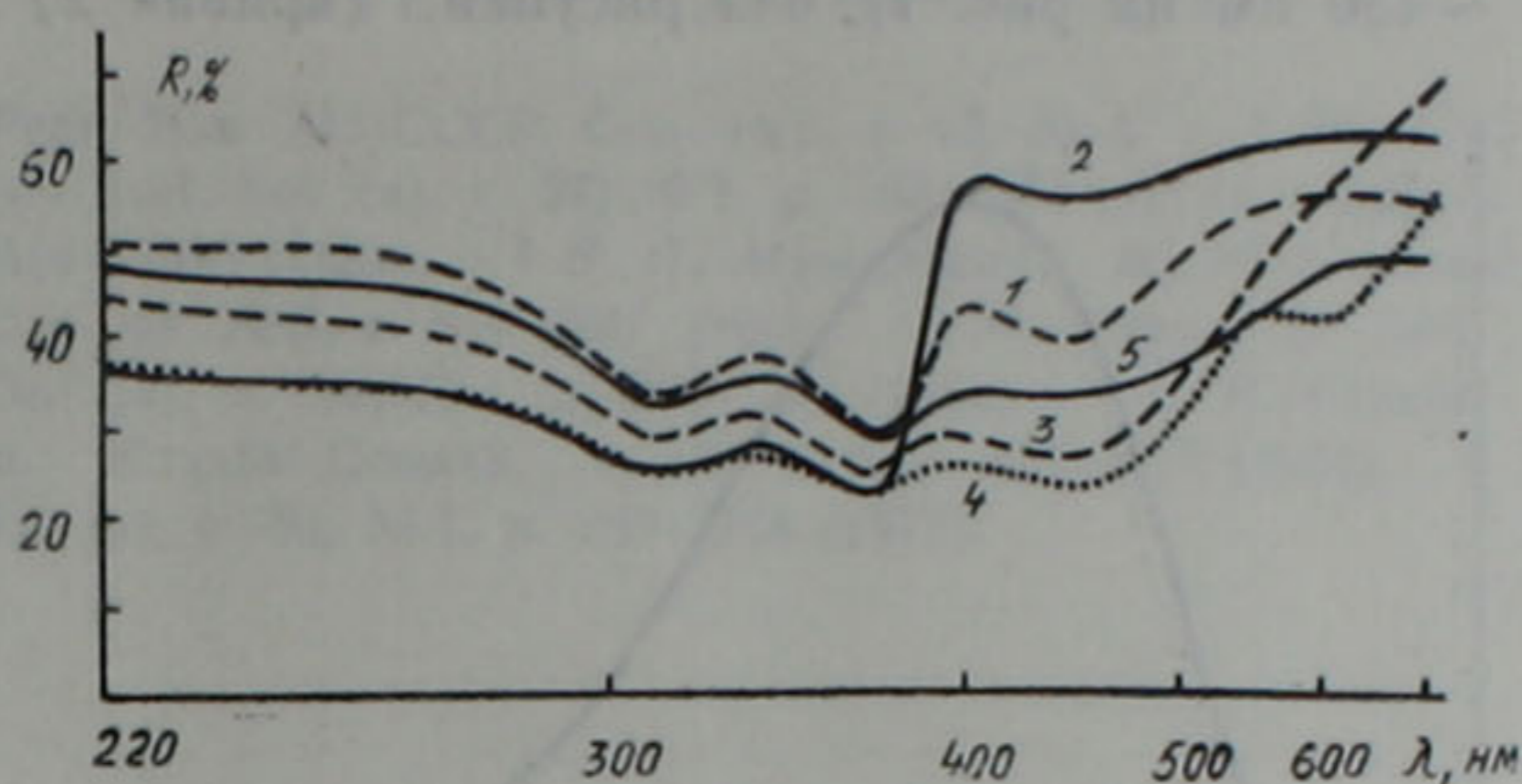
Рис. 2. Спектр зеленой люминесценции молибдата свинца с содержанием примеси 0,5 (1) и 1 мол. % CoO (2), 0,5 (3) и 5 мол. % Cr 2 O 3 (4), 1 мол. % V 2 O 5 (5)
